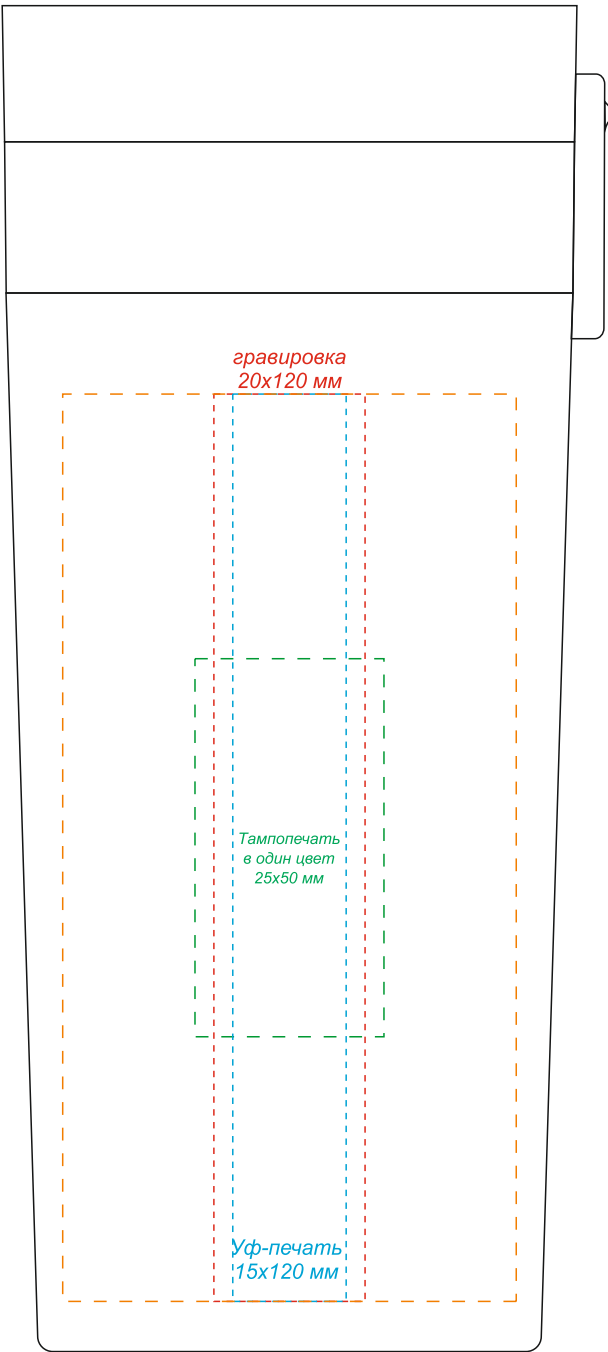
вид слева
